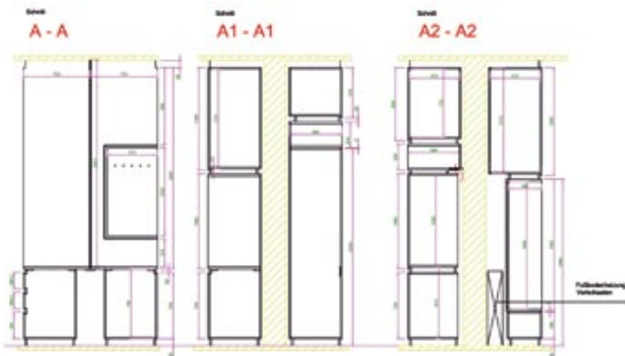
Die Schnitte zeigen, wie sich Küche und Garderobe in einem Block gegenüberstehen und teilweise durchdringen
